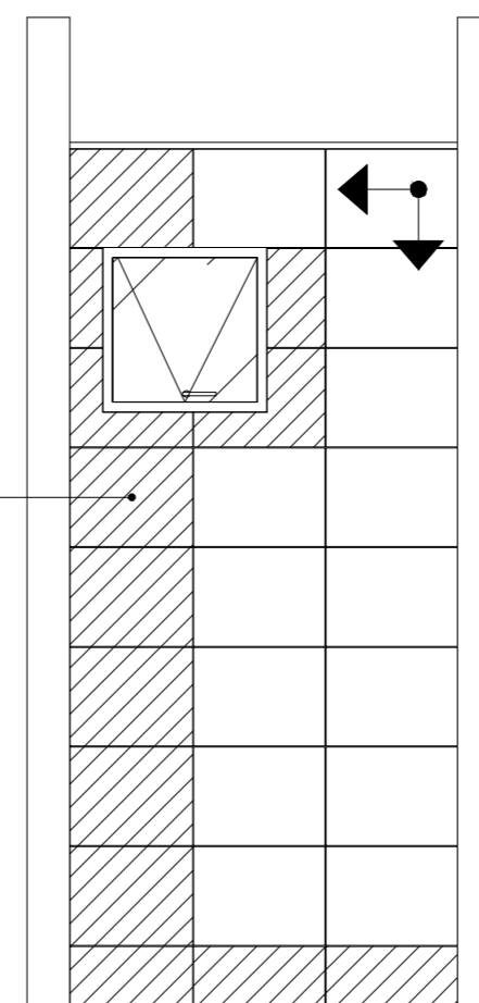
PAG. DE PAREDE - VISTA 02 Esc 1/25
