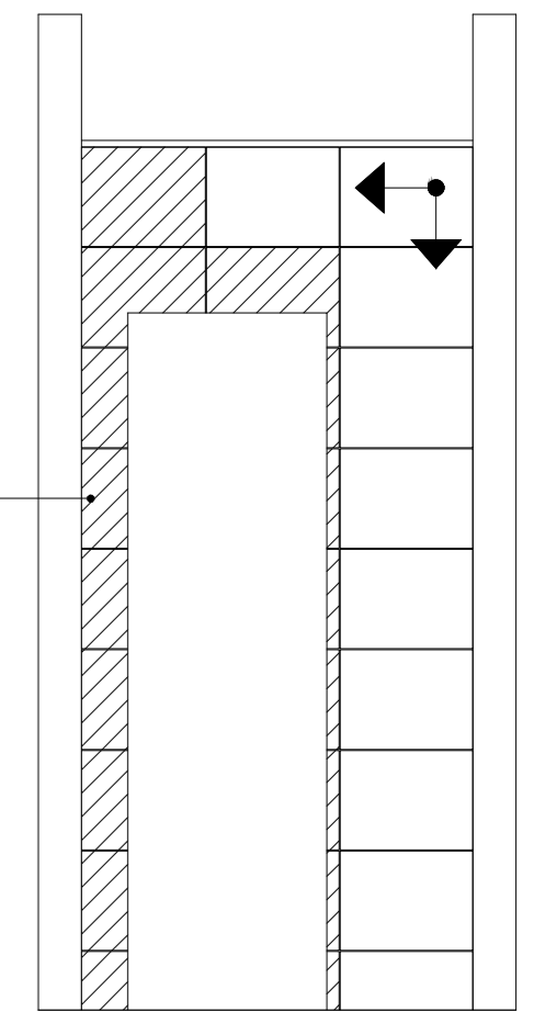
PAG. DE PAREDE - VISTA 04 Esc 1/25
