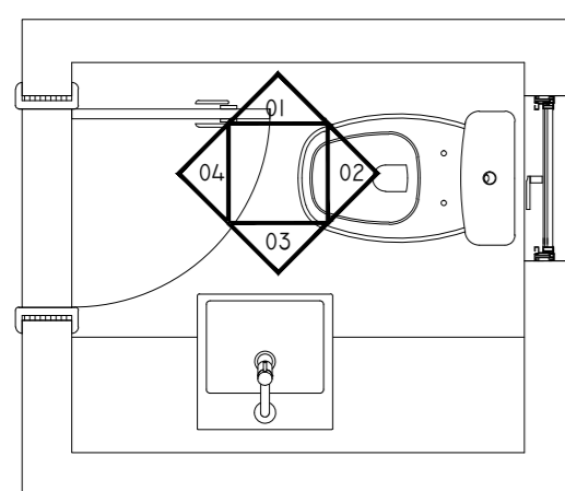
LAYOUT - Wc. FEM. Esc 1/25
